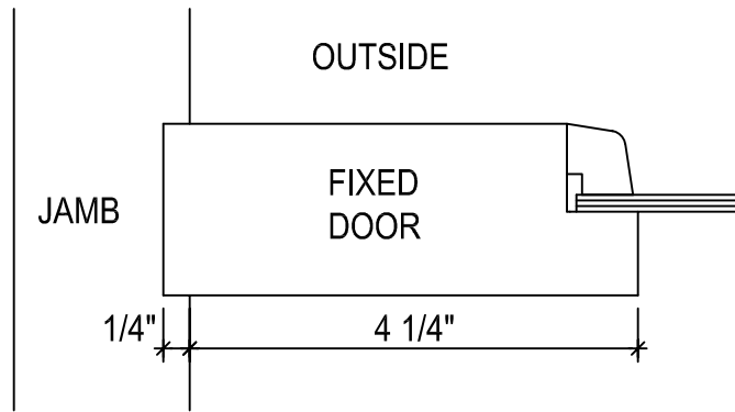
ⓑ FIXED DOOR
